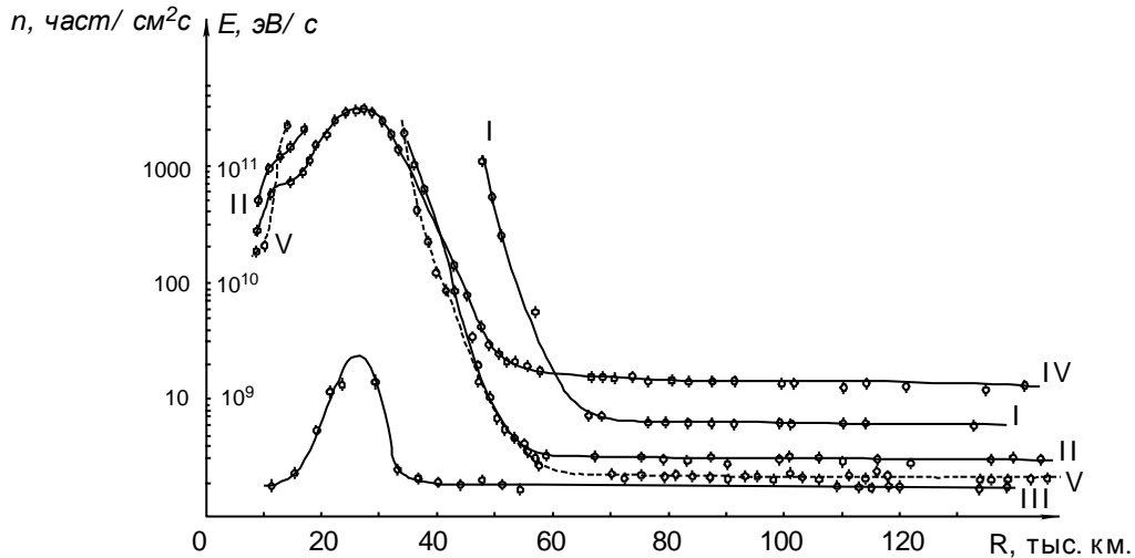
Рис. 8. Зависимость интенсивности от высоты полета первой космической ракеты.
