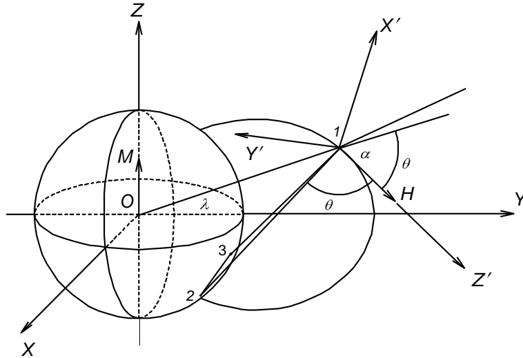
Рис. 18. К расчету инжекции частиц в точку 1 на данной силовой линии
