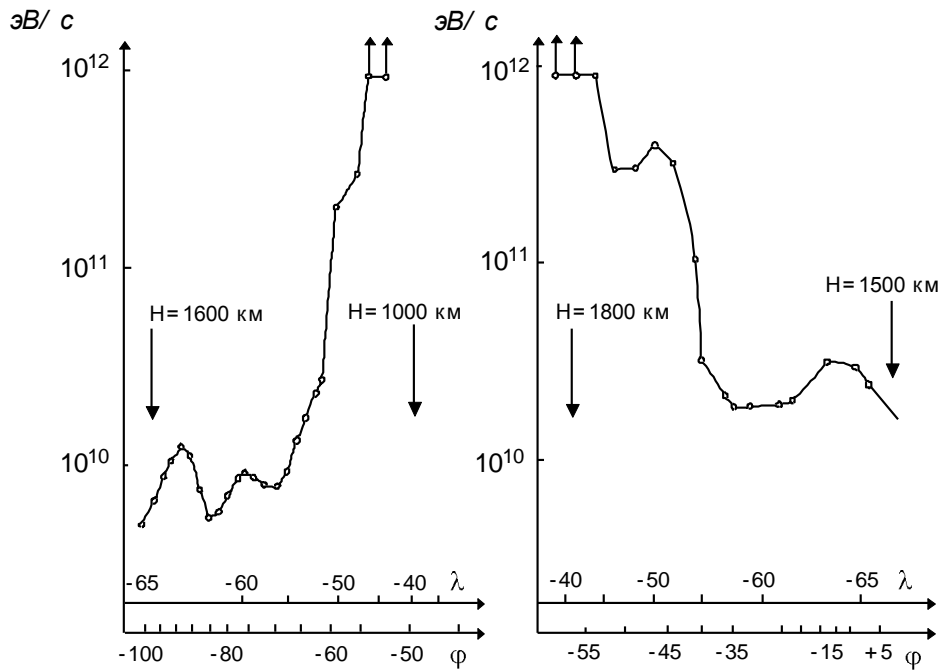
Рис. 10. Типичные образцы записей, выполненных в районе Южной Америки. По оси абсцисс - широта \lambda , долгота \varphi и высота H полета третьего спутника. По оси ординат - энергия, выделяемая в кристалле за 1 с, (ионизация по измерениям тока динода).
