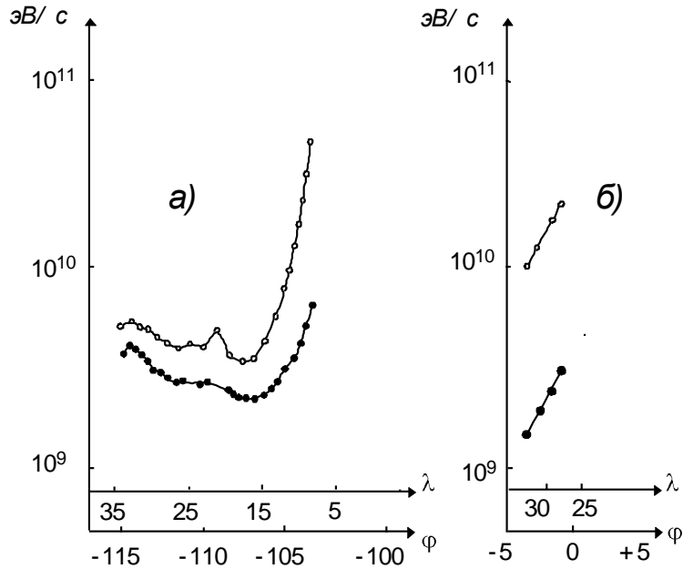
Рис. 14 Образцы записей, зафиксировавших вход третьего спутника во внутреннюю зону при движении с севера на юг.
