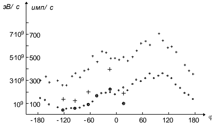
Рис. 12. Зависимость интенсивности фосфоресценции и темпа счета от положения орбиты третьего спутника относительно географических координат.
