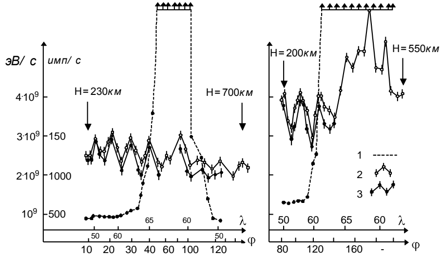
Рис. 4. Типичные примеры записи показаний сцинтилляционного счетчика в высоких широтах северного полушария.
