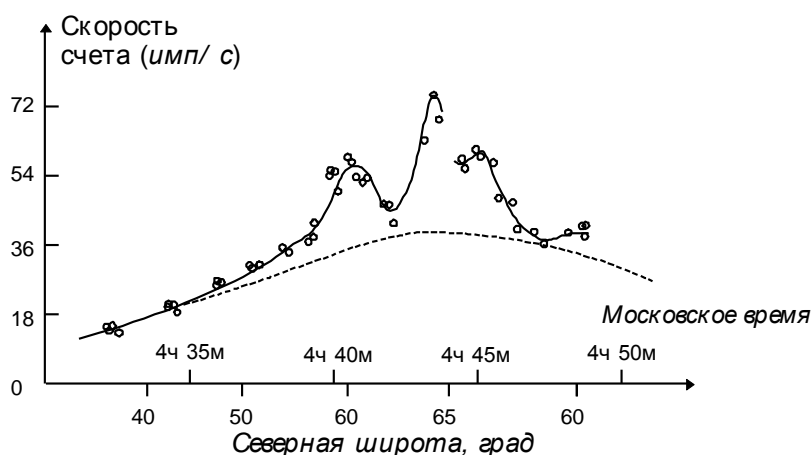
Рис. 3. Пример регистрации повышенной интенсивности в высоких широтах на втором спутнике 7.XI.57 г. Пунктир - обычный ход интенсивности.
