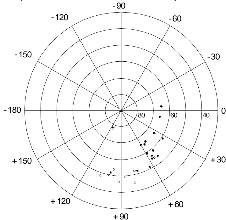
Рис. 6. Карта, показывающая места входа (кружки) и выхода (точки) третьего спутника из внешней зоны со стороны высоких широт в южном полушарии.
