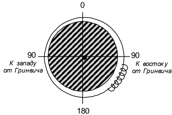
Рис. 13. Вероятное очертание нижней границы внутренней зоны в плоскости геомагнитного экватора.
