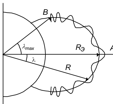
Рис. 16. Схематическое изображение движения заряженной частицы вдоль силовой линии магнитного поля Земли. R_{\text{э}} - расстояние до силовой линии в экваториальной плоскости, R - на широте \lambda , \lambda_{\text{max}} - максимальная широта, до которой может дойти частица.
