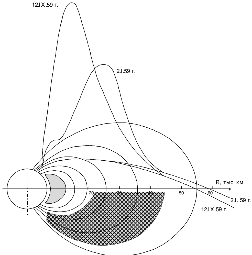
Рис. 7. Траектории первой и второй космических ракет в геомагнитных координатах.
