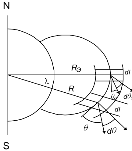
Рис. 17. К расчету числа частиц, образовавшихся в 1 с в трубке сечением 1 \text{ см}^2 на экваторе.
