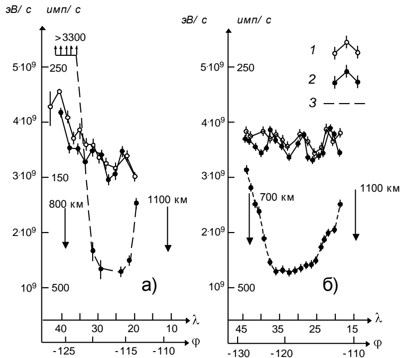
Рис. 15. Записи, показывающие выход из внешней зоны и подход к внутренней зоне в северном полушарии
