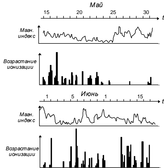
Рис. 9. Величина ионизационного эффекта во внешней зоне в северном полушарии за период с 15.V по 17.VI.58 г. и всемирный магнитный индекс (по трехчасовым интервалам) за то же время.
