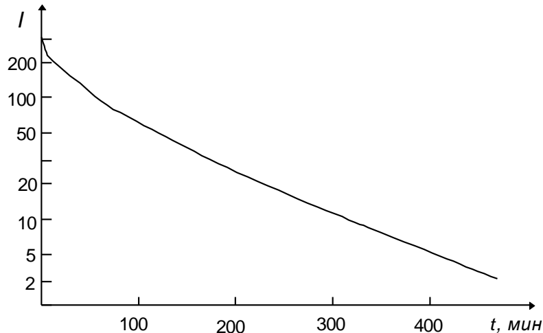
Рис. 11. Зависимость интенсивности фосфоресценции кристалла йодистого натрия от времени после облучения.
