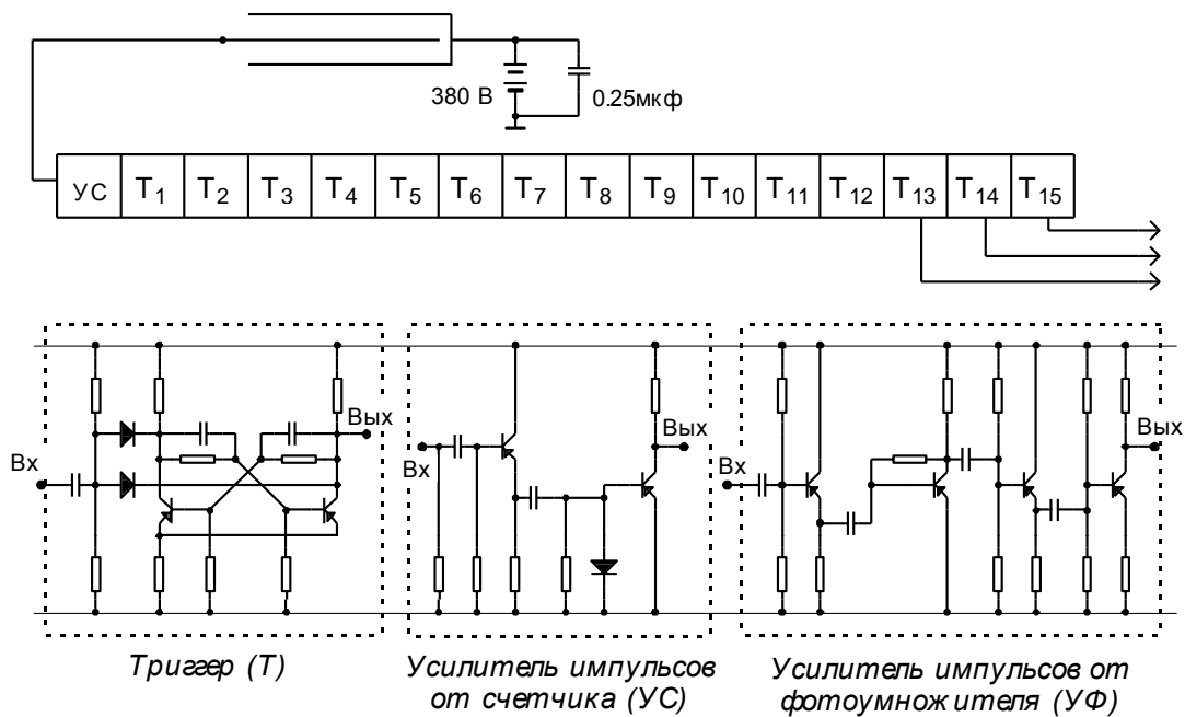
Рис. 2. Блок-схема газоразрядного счетчика и принципиальная схема типовых элементов электроники.
