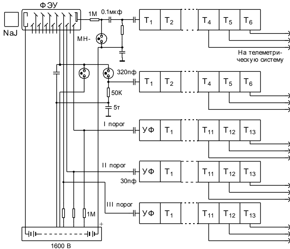
Рис. 1. Блок-схема сцинтилляционного счетчика.
